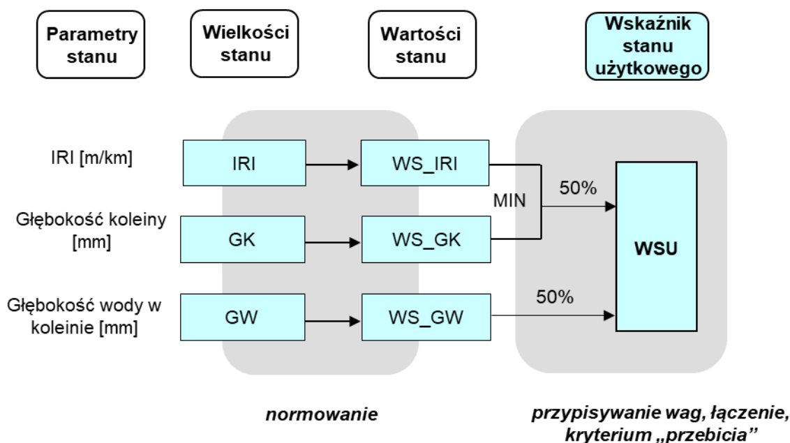
Rysunek 20: Schemat wyznaczenia wskaźników zespolonych w wariantcie podstawowym
