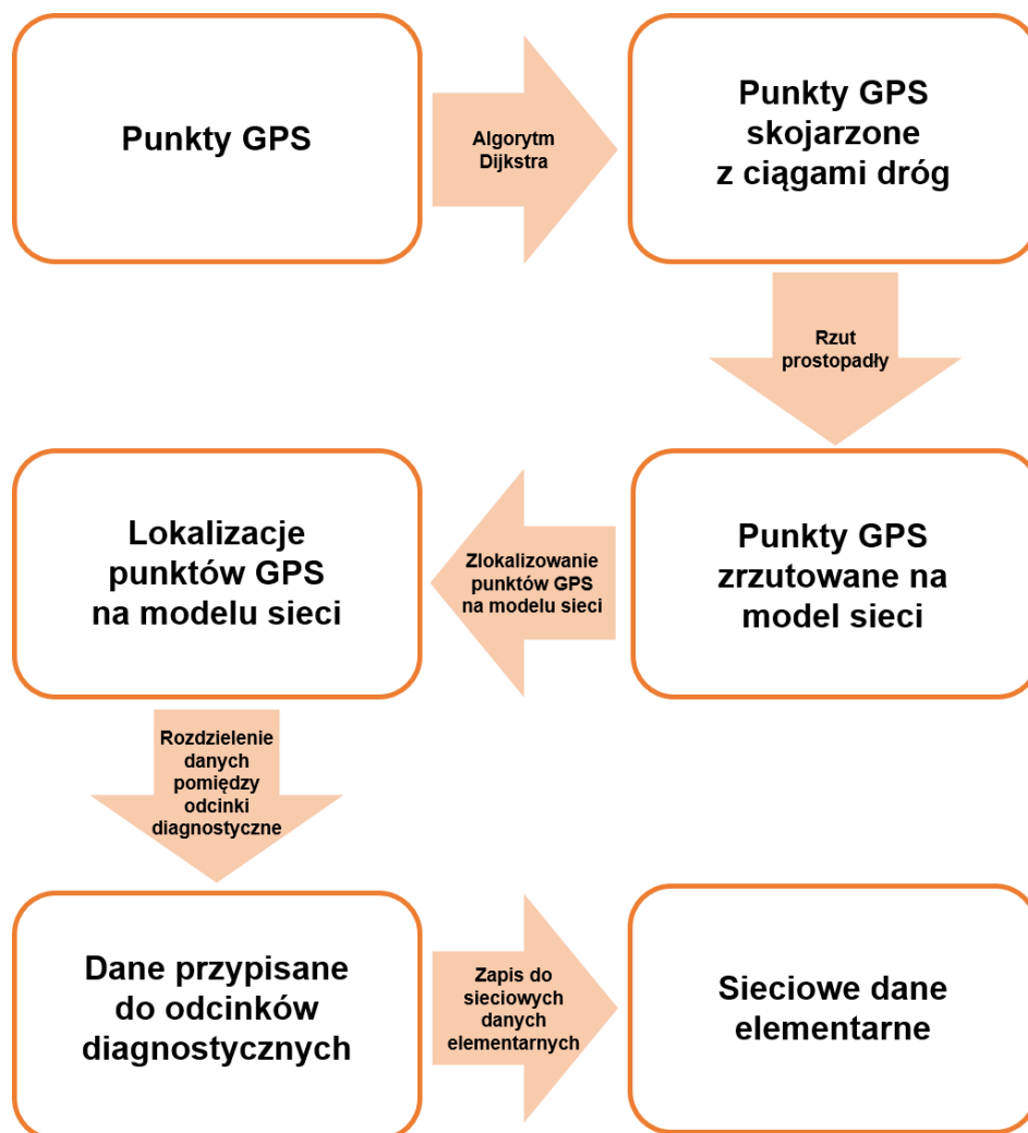
Rysunek 4: Schemat przebiegu procedury projekcji
