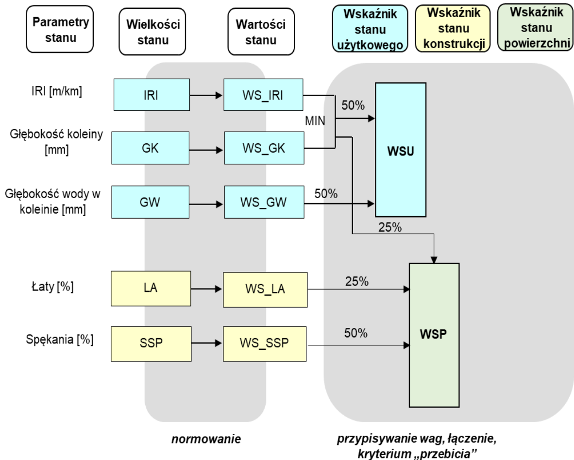
Rysunek 21: Schemat wyznaczania wskaźników zespolonych w wariantie zalecany
