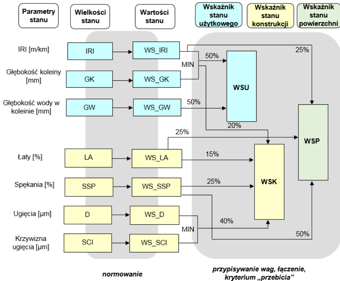
Rysunek 22: Schemat wyznaczania wskaźników zespolonych w wariantcie optymalnym
