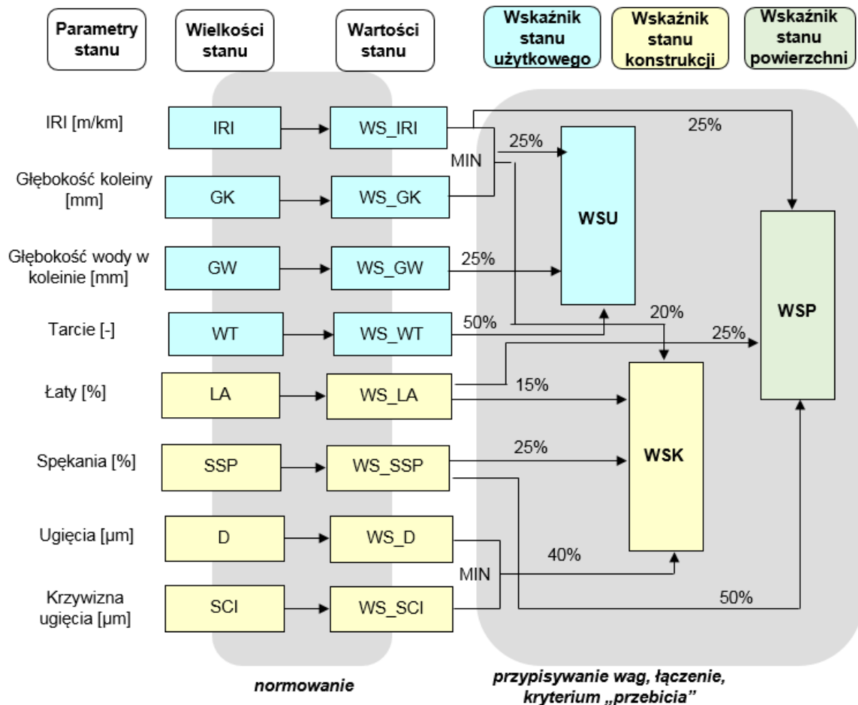
Rysunek 23: Schemat wyznaczania wskaźników zespolonych w wariacie optymalnym uzupełnionym o badanie właściwości przeciwpoślizgowych
