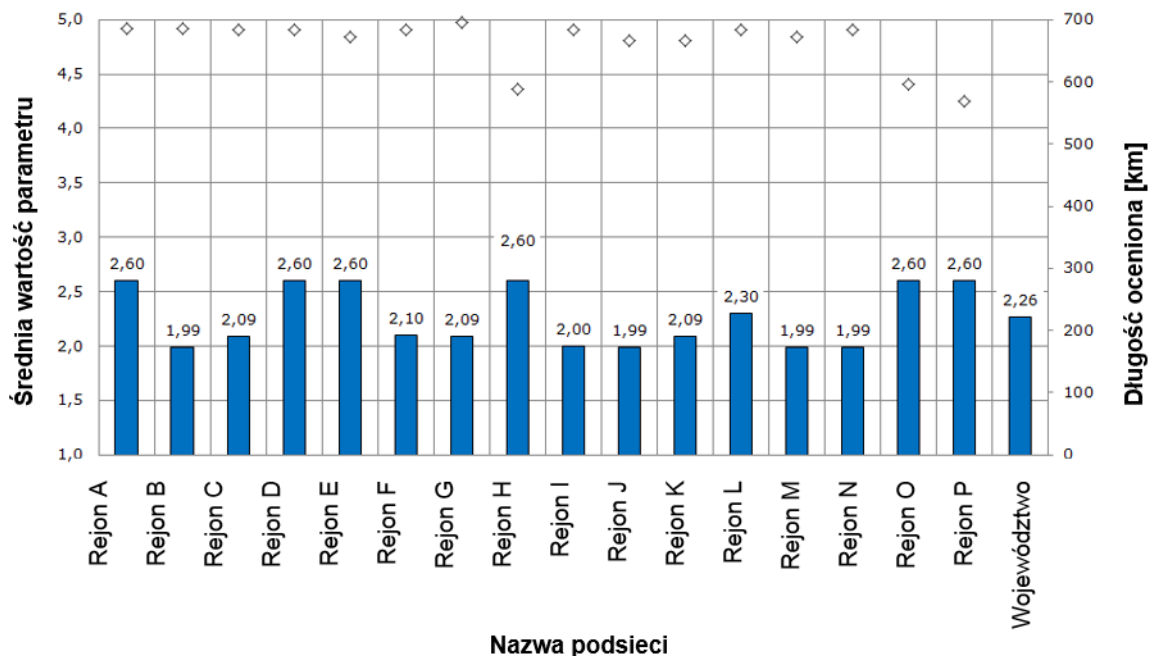
Rysunek 44: Przykład wykresu słupkowego ze średnimi wartości parametru stanu (dane fikcyjne)
