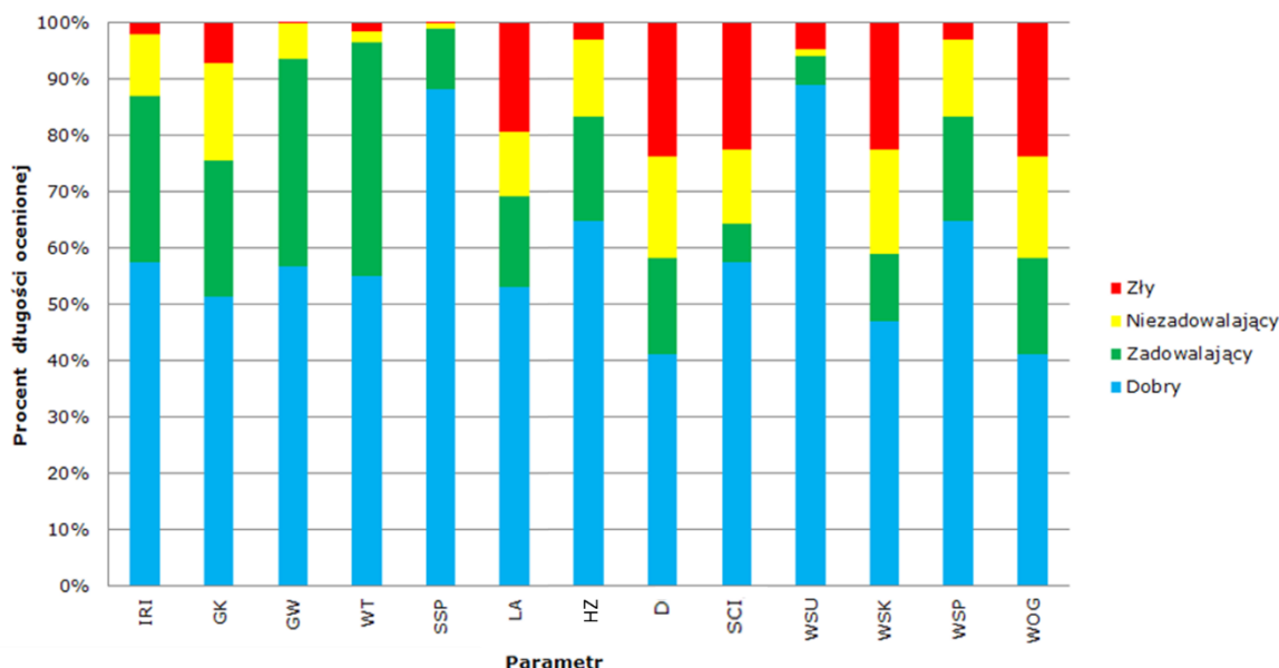
Rysunek 27: Przykład wykresu słupkowego z rozkładem częstości klas stanu (dane fikcyjne)
