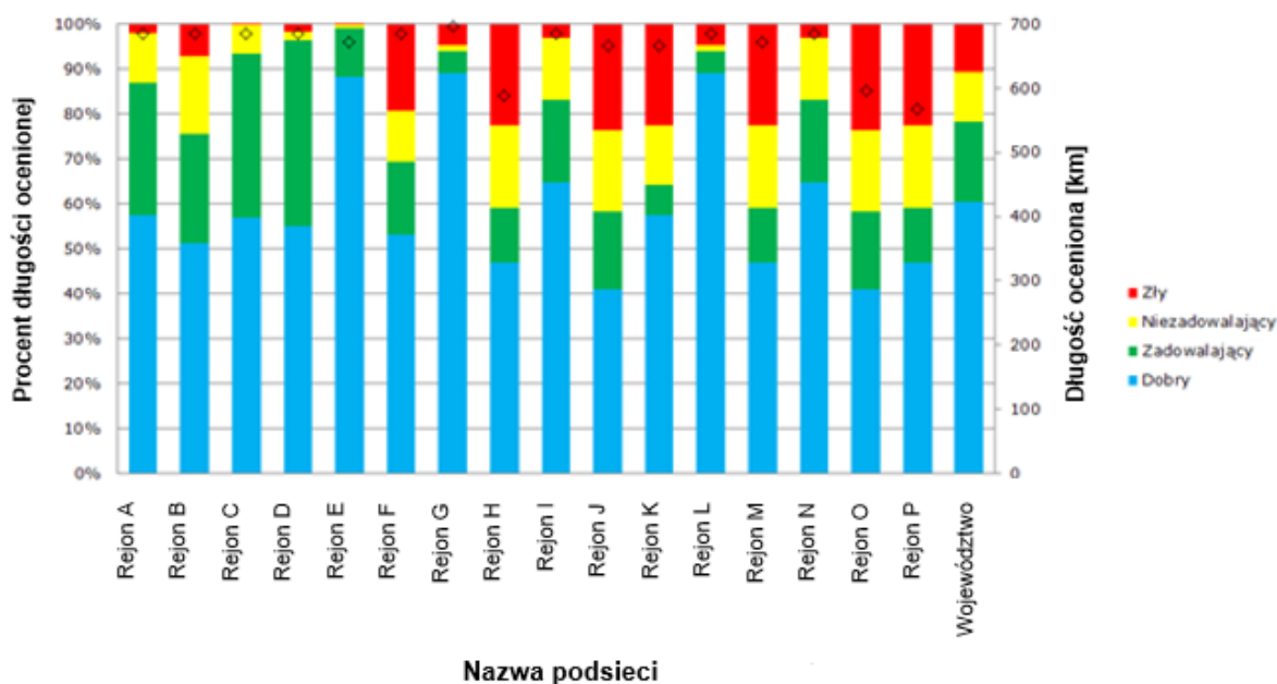
Rysunek 46: Przykład wykresu słupkowego z rozkładem częstości klas stanu
