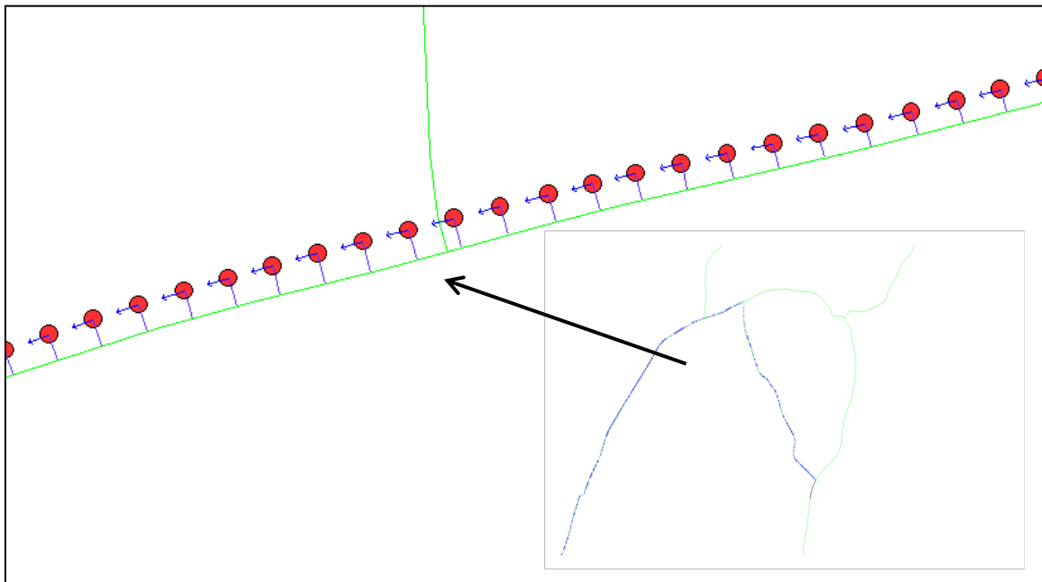
Rysunek 6: Ilustracja rzutu prostopadłego punktów pomiarowych na łamane modelu sieci, czerwone punkty oznaczają lokalizacje punktów pomiarowych
